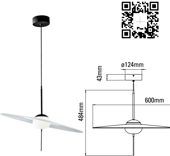
MONO L600
